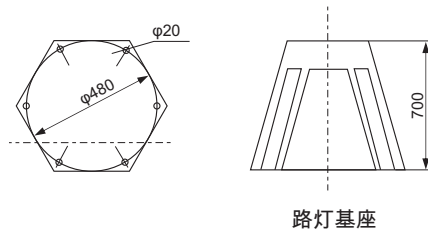
路灯基座
