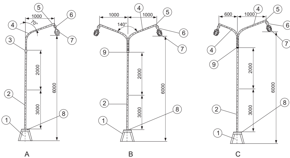
BAM52-10A□□ 配装灯具示意图
